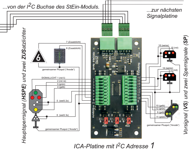
ICA-Platine mit I 2 C Adresse 1
