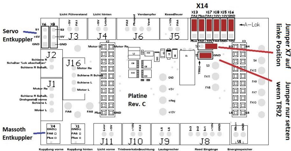
Platine LOKPLSHMAL im Auslieferungszustand
