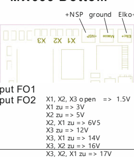
MX635 Bottom
