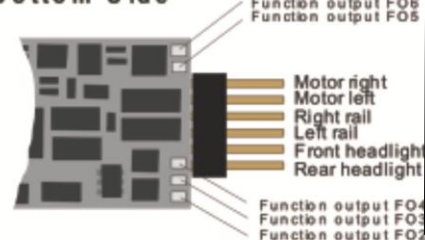
Bottom Side
