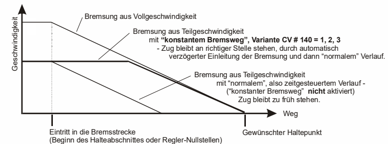
Erste Variante für konstanten Bremsweg
